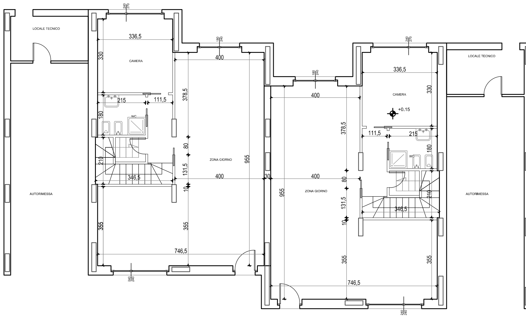
PIANO TERRENO - scala 1:100
